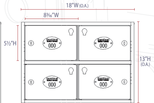
4 DOOR REGULAR INSERT
