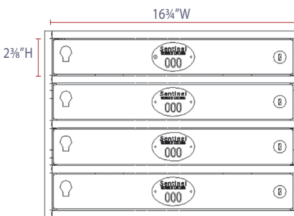
4 DOOR HORIZONTAL INSERT
